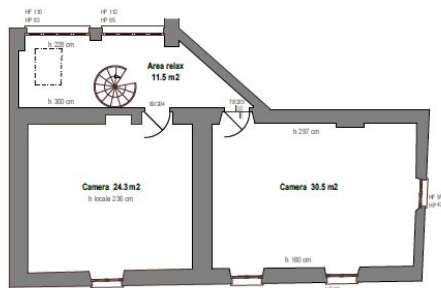
Piano mansardato - superficie di piano 89 m 2
