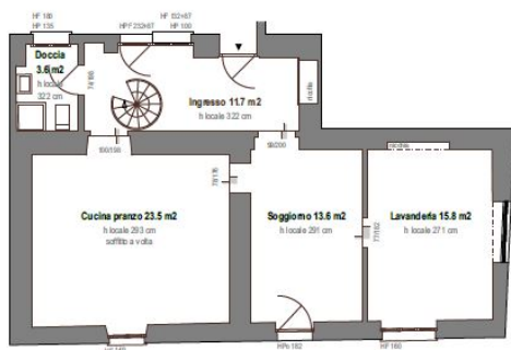
Piano terreno - superficie di piano lorda 93 m 2
