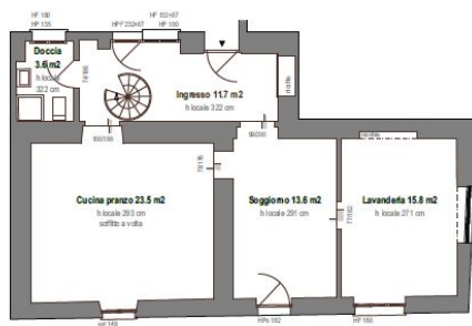
Piano terreno - superficie di piano lorda 93 m 2
