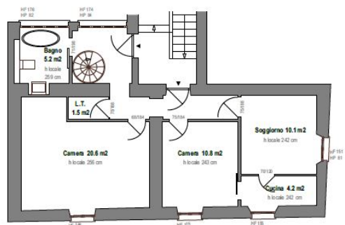
Piano primo - superficie di piano lorda 85 m 2
